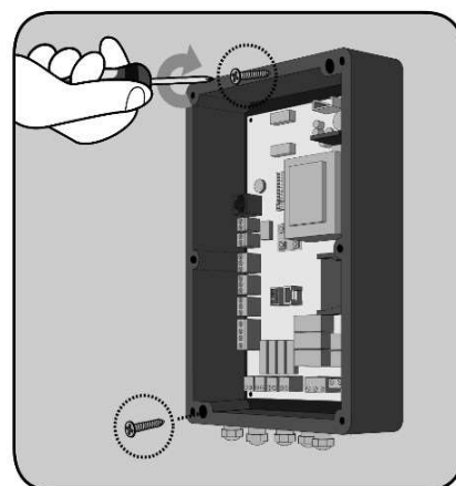
GEHÄUSE AN DER WAND BEFESTIGEN
