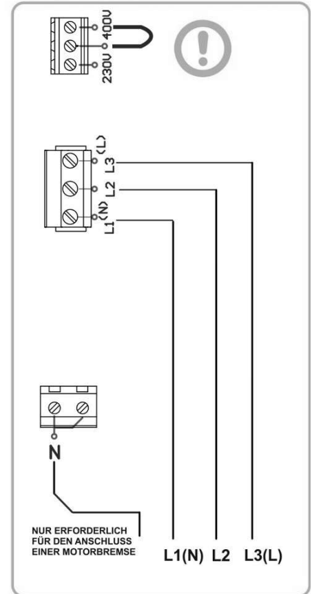
SPANNUNGSVERSORGUNG 400V DREHSTROM
